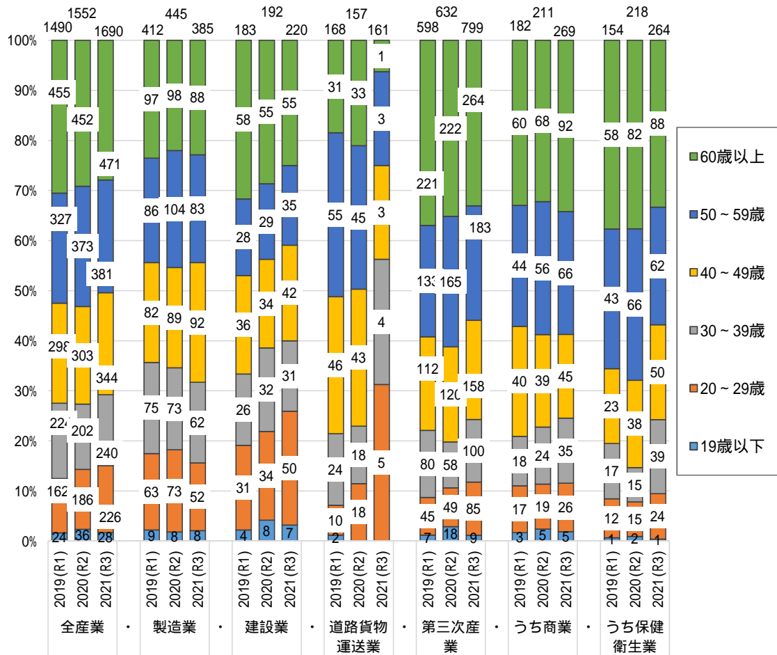
主要業種・年齢階層別労働災害発生割合 (休業4日以上 2019~2021 数値は人数 愛媛労働局)
