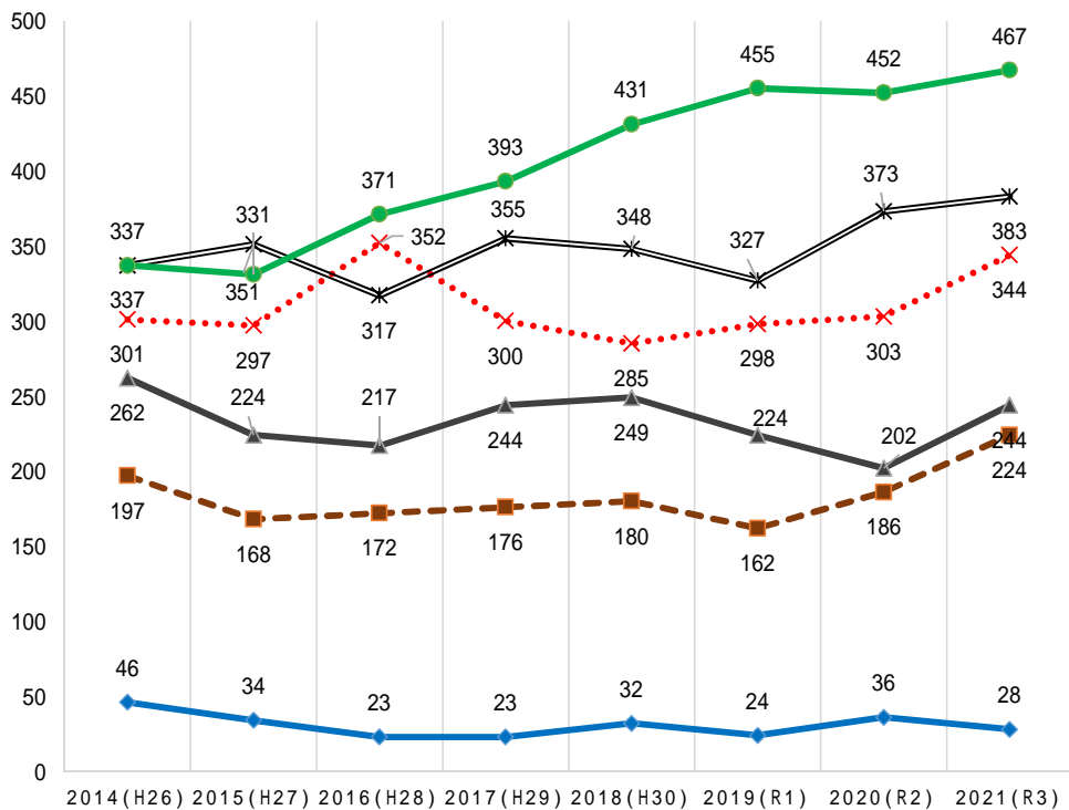
年齢階層別死傷者数の推移 (休業4日以上 2014~2021 (R3) 愛媛労働局)
