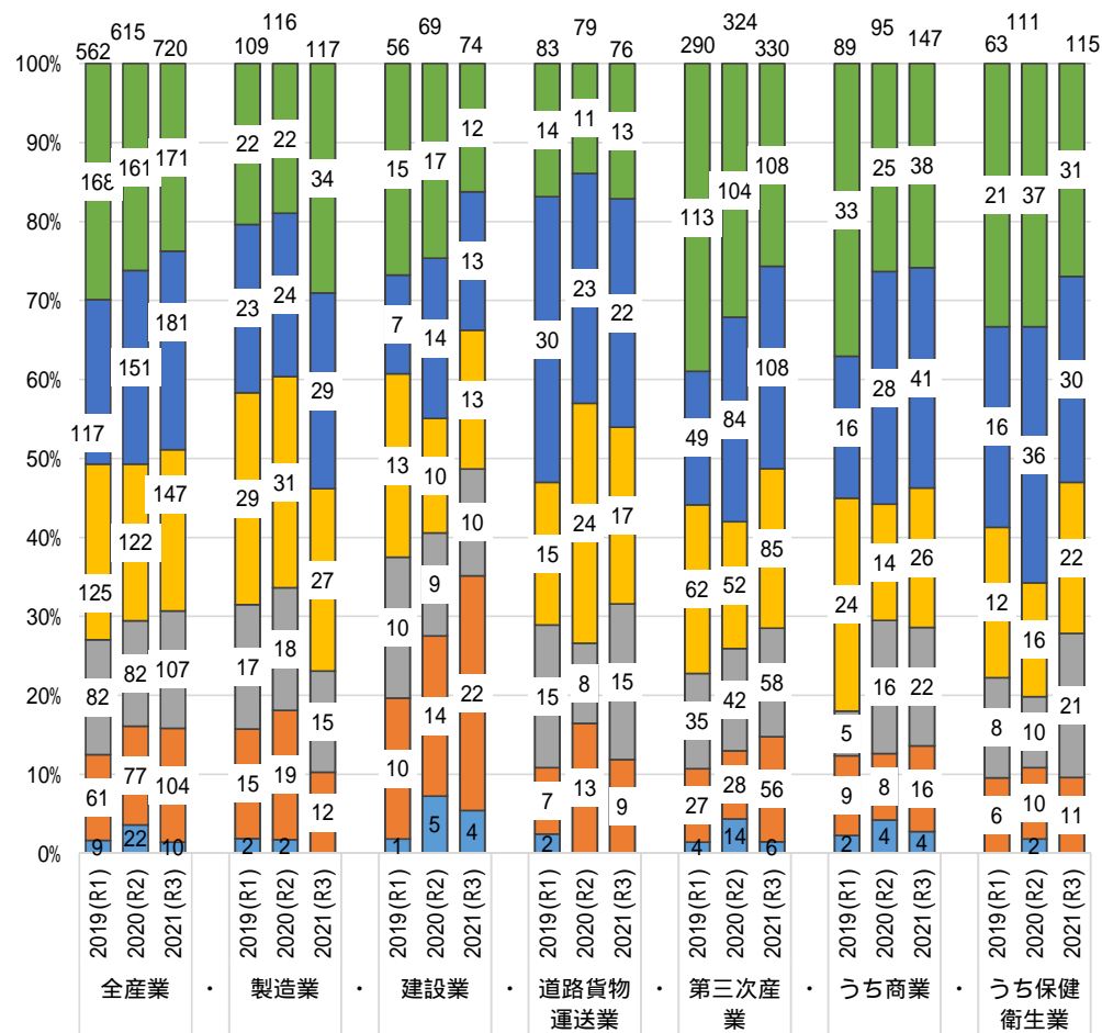
主要業種・年齢階層別労働災害発生割合 (休業4日以上 2019~2021 数値は人数 松山署)
