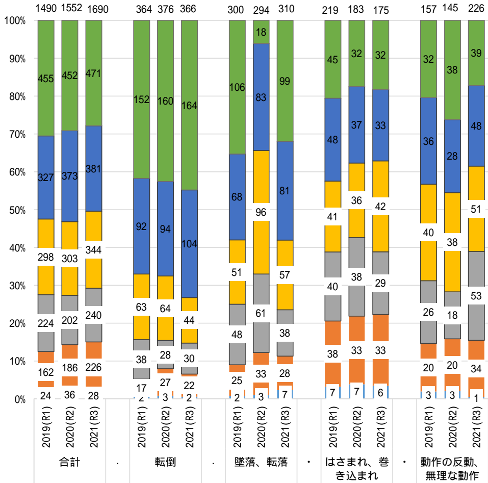
主要事故の型・年齢階層別労働災害発生割合 (休業4日以上 2019~2021 数値は人数 愛媛労働局)
