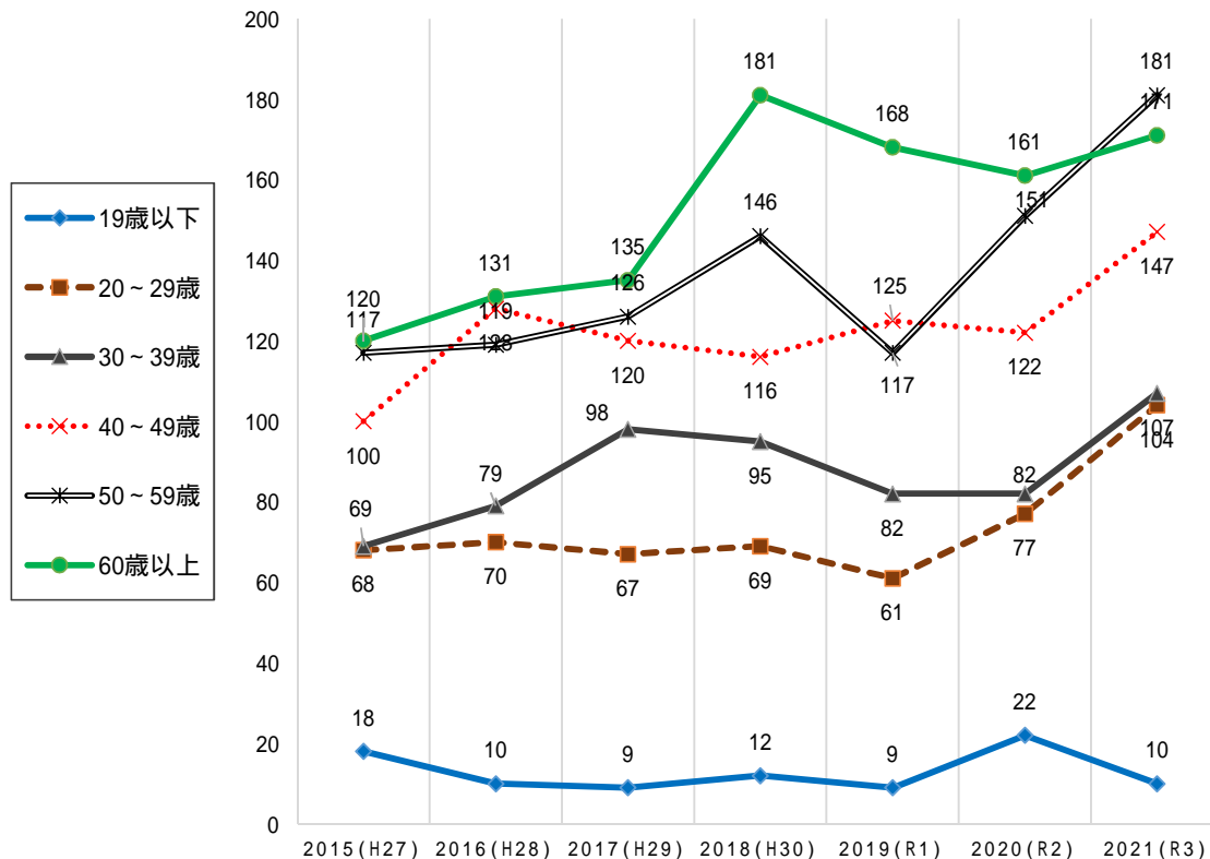
年齢階層別死傷者数の推移 (休業4日以上 2017(H27)~2021 (R3) 松山署)
