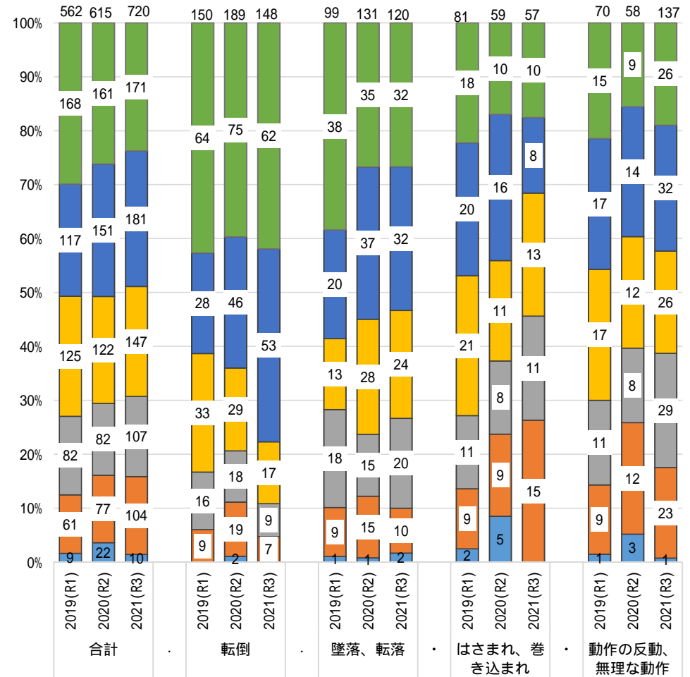
主要事故の型・年齢階層別労働災害発生割合 (休業4日以上 2019~2021 数値は人数 松山署)
